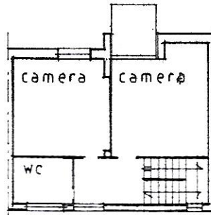
PIANO P.RIMO h=2,80
